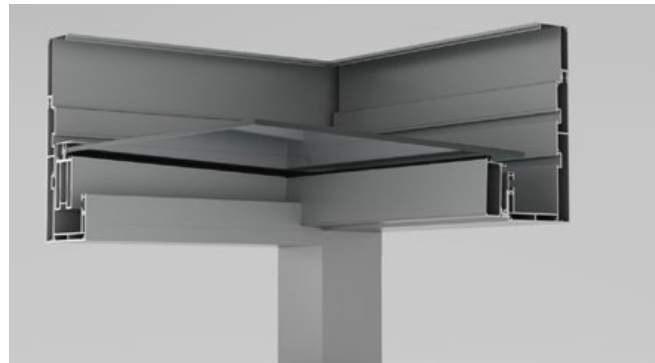
Taras z płaskim dachem Widok rynny
