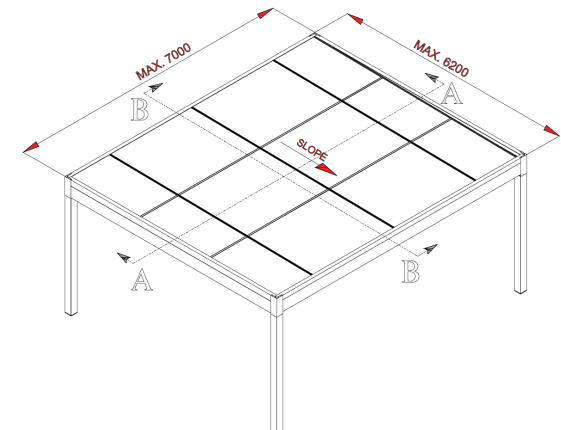
Taras z płaskim dachem Maksymalne wymiary
