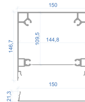
Słupek Wymiary
