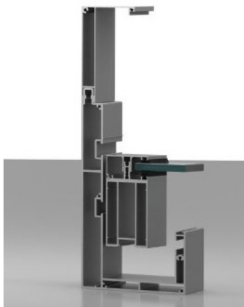
Taras z płaskim dachem Widok rynny
