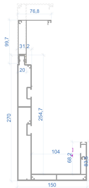
Rynna Wymiary
