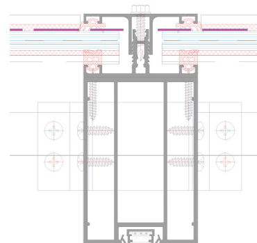
Krokiew Wymiary
