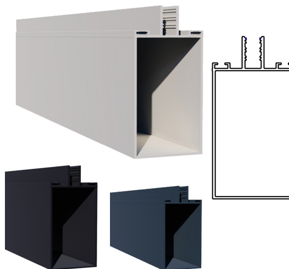
V001007 Krokiew
